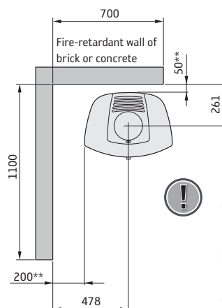
Fire-retardant wall of brick or concrete - негорючая стена из кирпича или бетона
