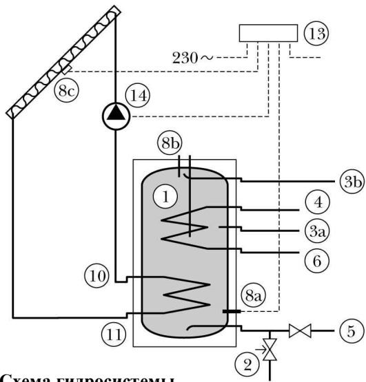
Схема гидросистемы
